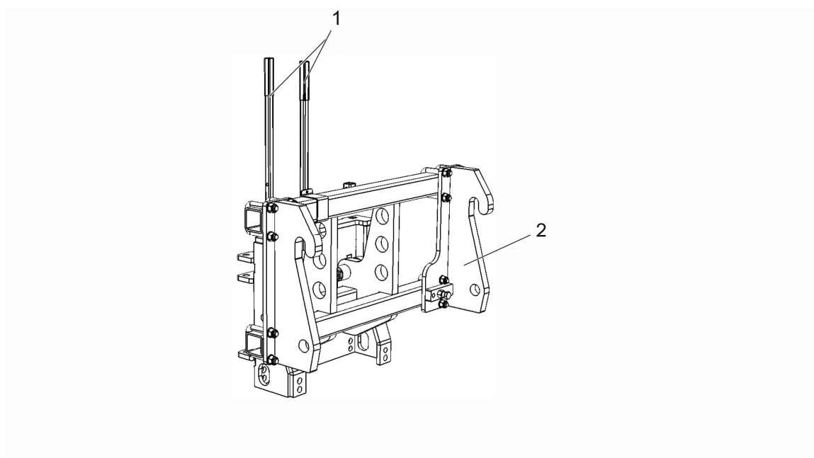
Illustration 4 Eftermonteringssystem med pejlestok
