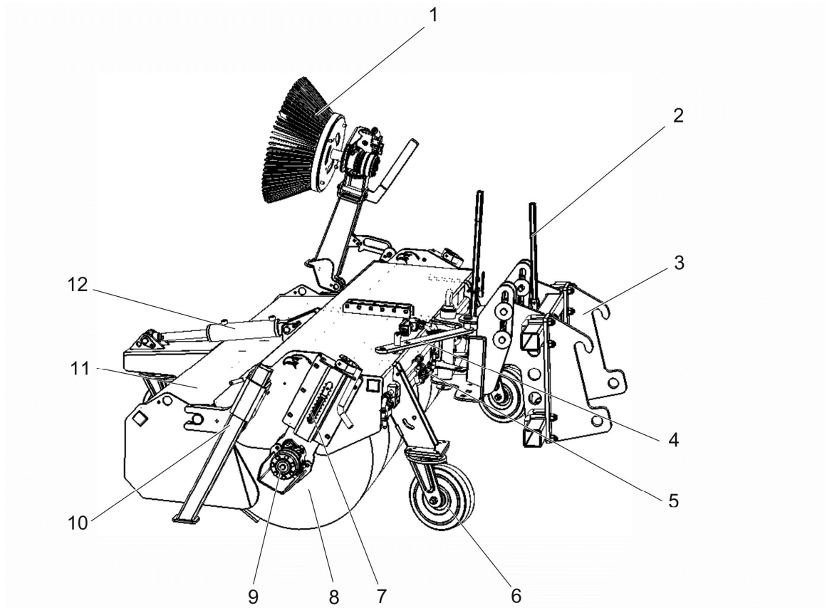
Illustration 3 Fejemaskine K 600 fuldt udstyret
