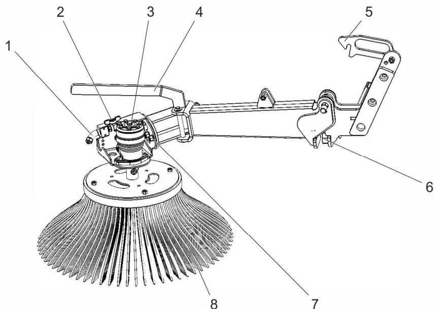
Illustration 16 Indstilling og fastlåsning af sidekosten
