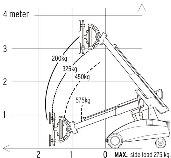
WINLET 575 MAX. LOAD kg.
