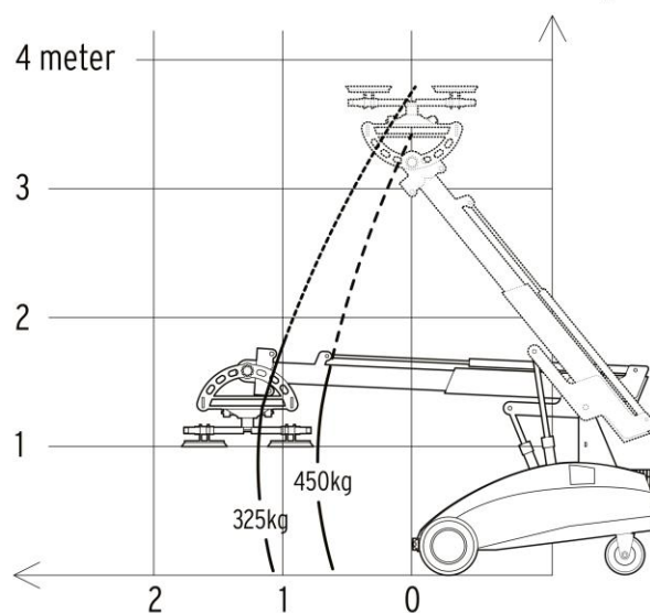
WINLET 575 MAX. LOAD/REACH kg.
