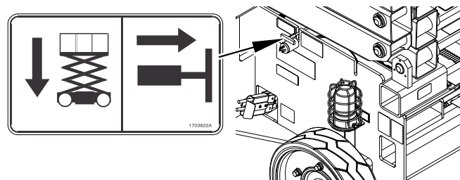
Placering af T-håndtag til manuel sænkning
