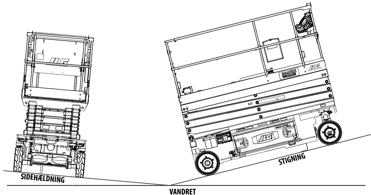
Figur 3-2. Stigning og sidehældning – Kørsel – Platform i opbevaringsposition
