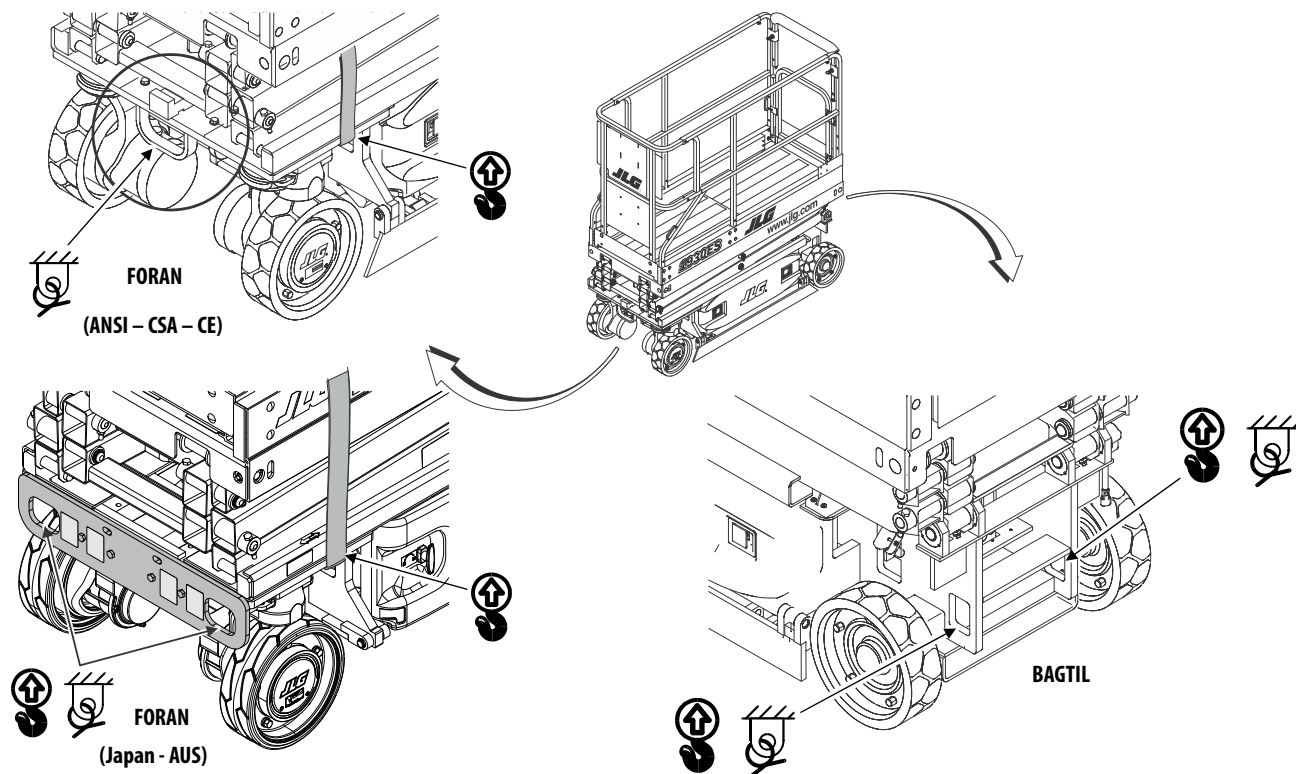
Figur 3-4. Diagram over løftning og fastspænding
