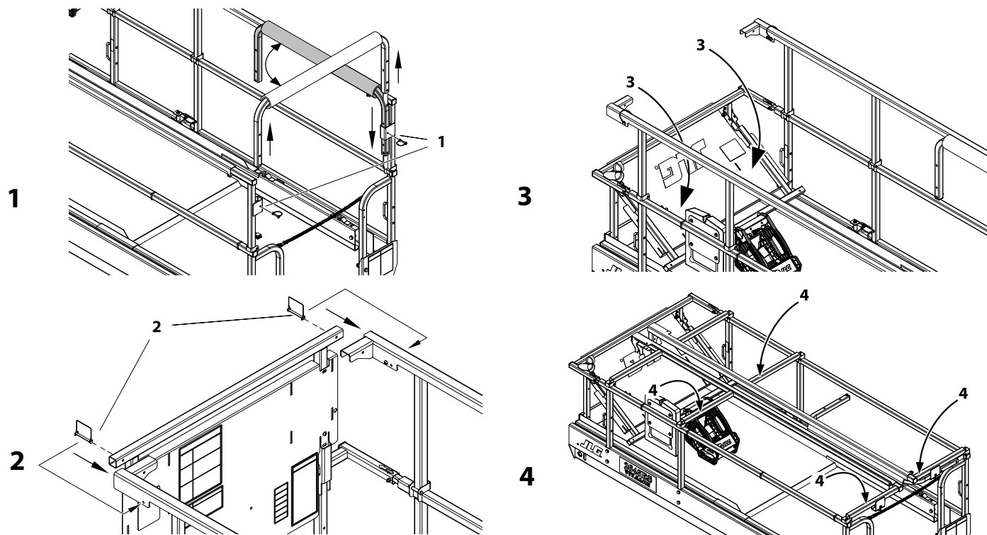
Figur 3-3. Platformens gelændere – Nedfoldningssekvens
