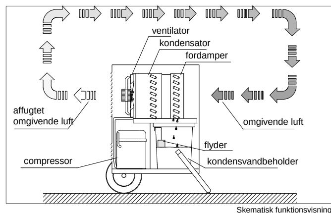
Skematisk funktionsvisning
