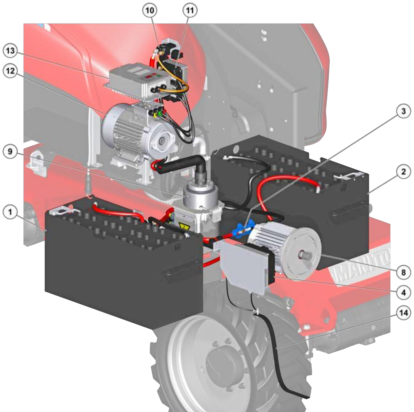
Figur 179: Kontrol af de elektriske højspændingsforbindelsers tilspænding 1 - 160 ATJE RC S1 - 180 ATJE RC S1 - anden version
