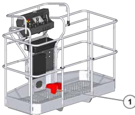
Figur 62: Fodkontakt
