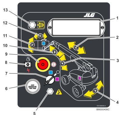
Figur 10. 860SJ med undervognsstyrepanel MMSO og DPF
