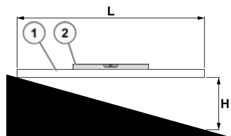
Figur 89: Hældningsmåling
