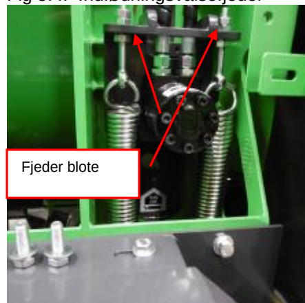
Fig 5.4. Indfødningsvalsefjeder
