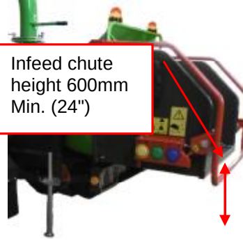
Fig 3.4.3 Indfødningsstragt højde
