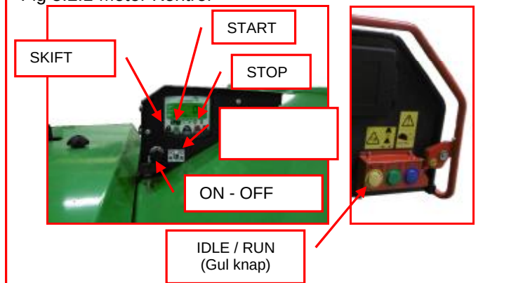
Fig 5.2.1 Motor Kontrol
