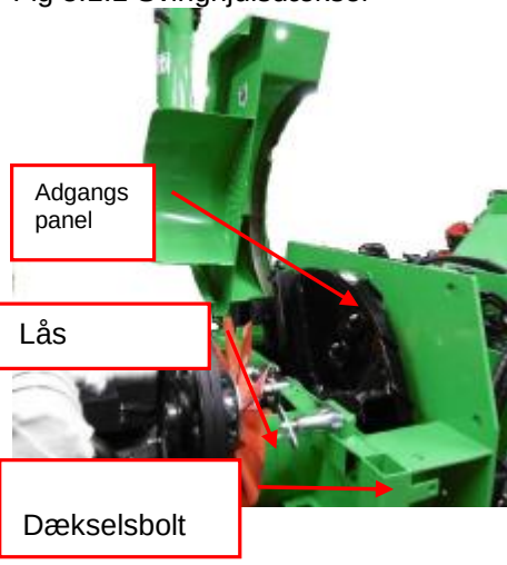
Fig 5.1.1 Svinghjulsdæksel
